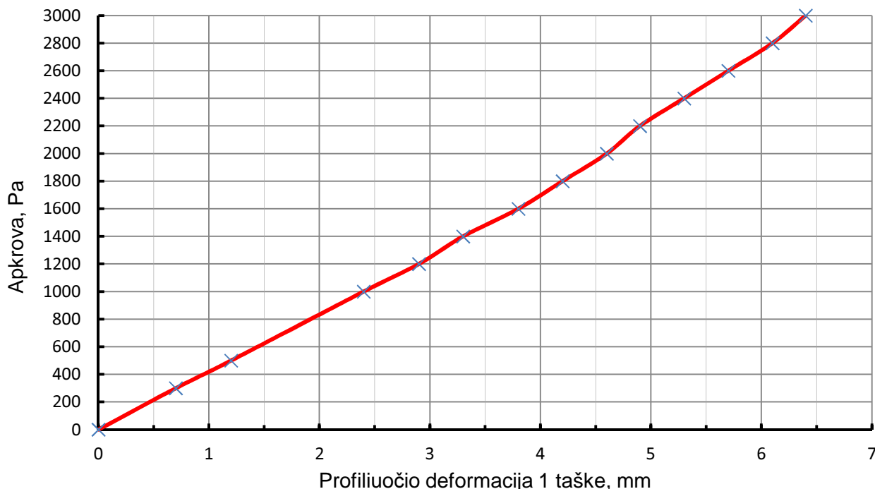
1 paveikslas. Vertikalaus profiliuočio apkrovos-deformacijos kreivė
