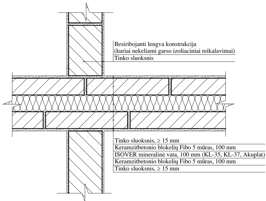
4 pav. Vidinės atitvaros, kuriai keliami oro garso izoliacijos reikalavimai ir vidinės atitvaros, kuriai nekeliama oro garso izoliaciniai reikalavimai, jungimo mazgas
