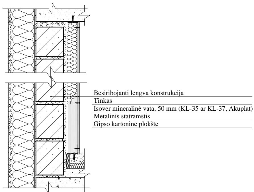
1 pav. Apdaro sluoksnio įrengimas ant besiribojančios lengvos konstrukcijos (vertikalus pjūvis)
