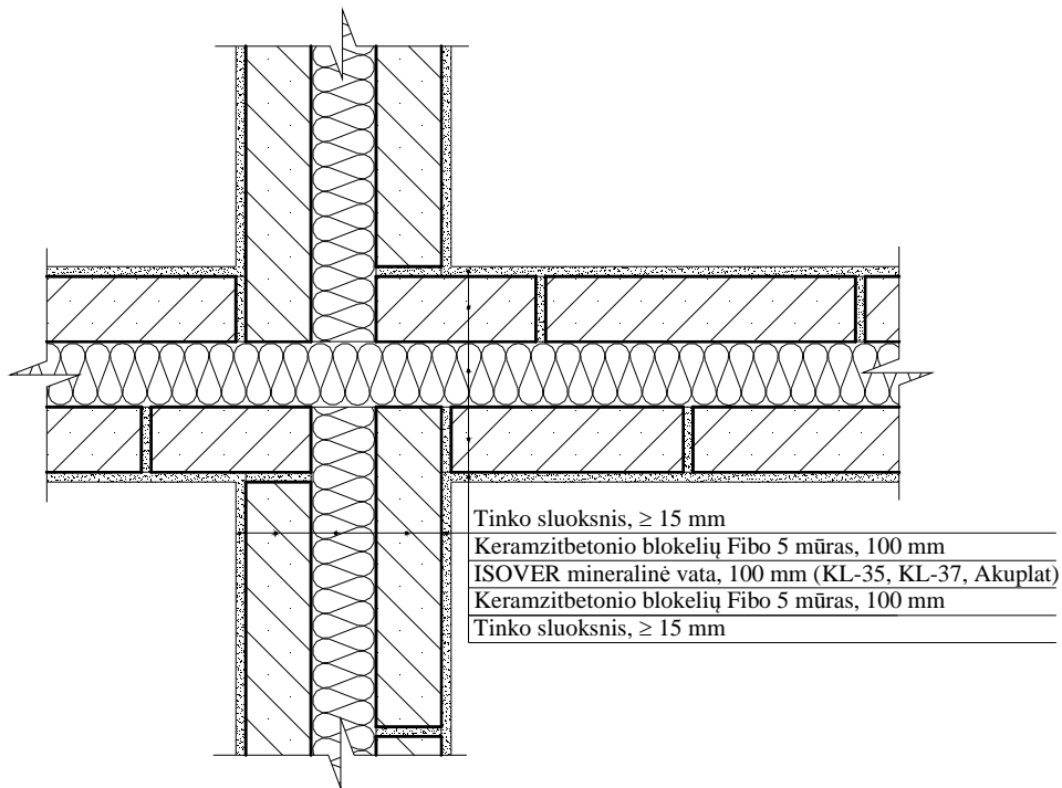
3 pav. Dviejų besikertančių vidinių atitvarų jungimo mazgas
