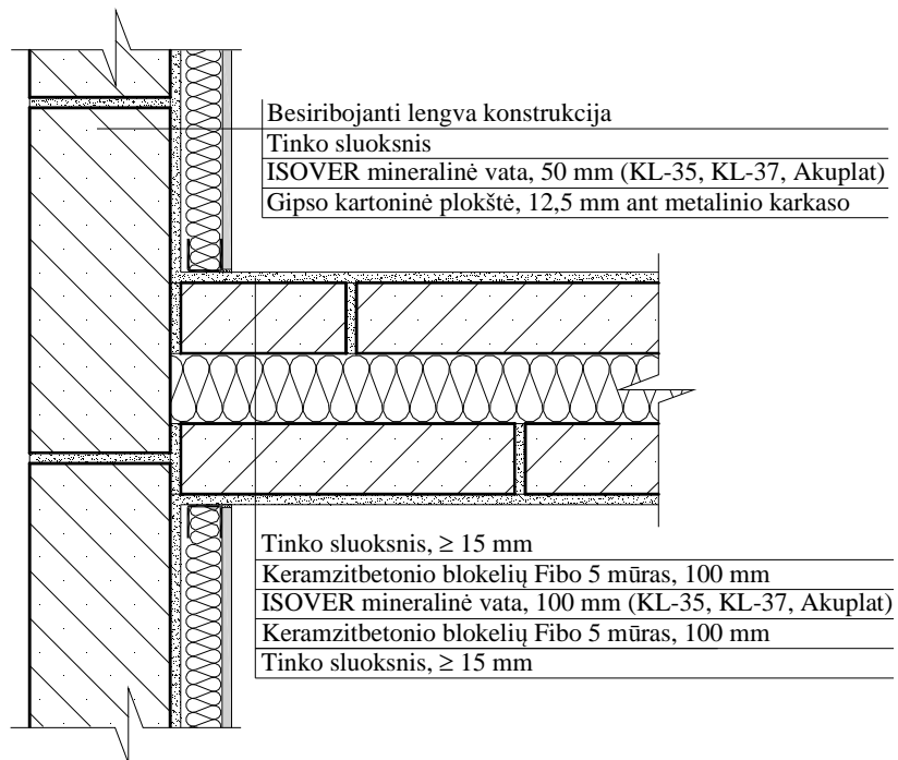
2 pav. Jungtis su lengva besiribojančia konstrukcija – ant besiribojančios konstrukcijos įrengtas apdaras
