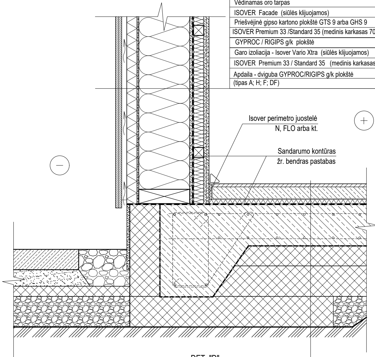
DET. "D"
