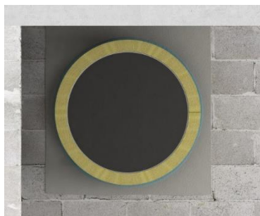
5.5 pav. Ortakio izoliavimas kai atstumas iki konstrukcijos \leq 200\text{mm} ir daugiau nei izoliacijos storis
