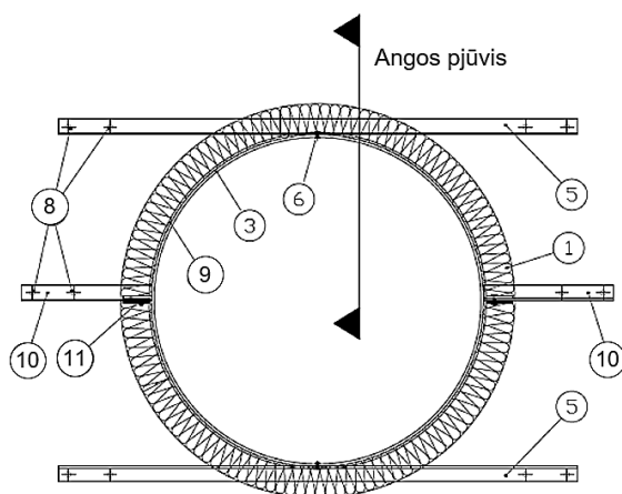
5.1 pav. Angos įrengimas, principinis brėžinys
