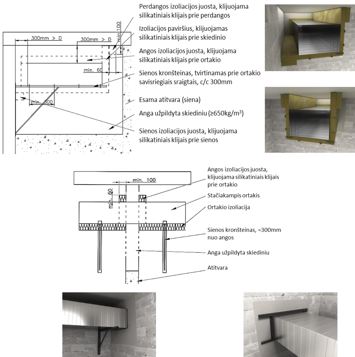
6.9 pav. Stačiakampių ortakio ir angos įrengimas arti atitvarinių konstrukcijų, principiniai brėžiniai
