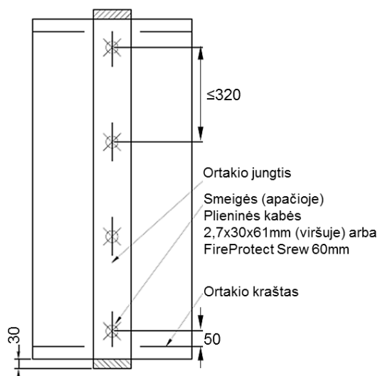
a) ortakio viršaus ir apačios izoliavimas
