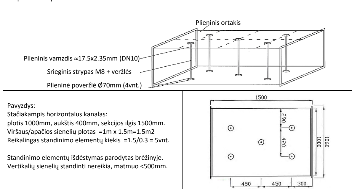
7.1pav. Principinė standinimo schema
