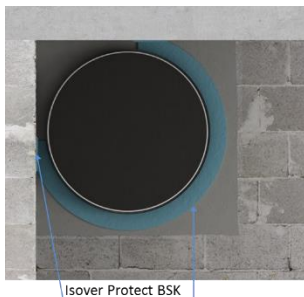
5.6 pav. Ortakio izoliavimas, kai atstumas iki konstrukcijos mažesnis nei izoliacijos storis
