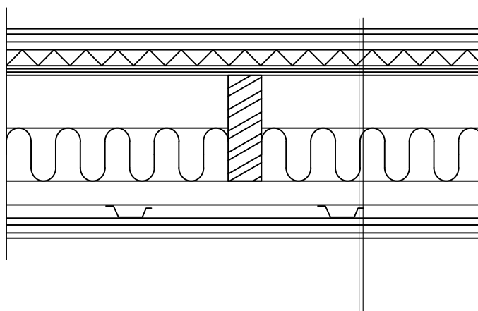
DET. "MP-5"
