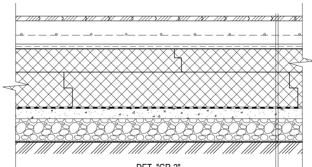
DET. "GR-2"
