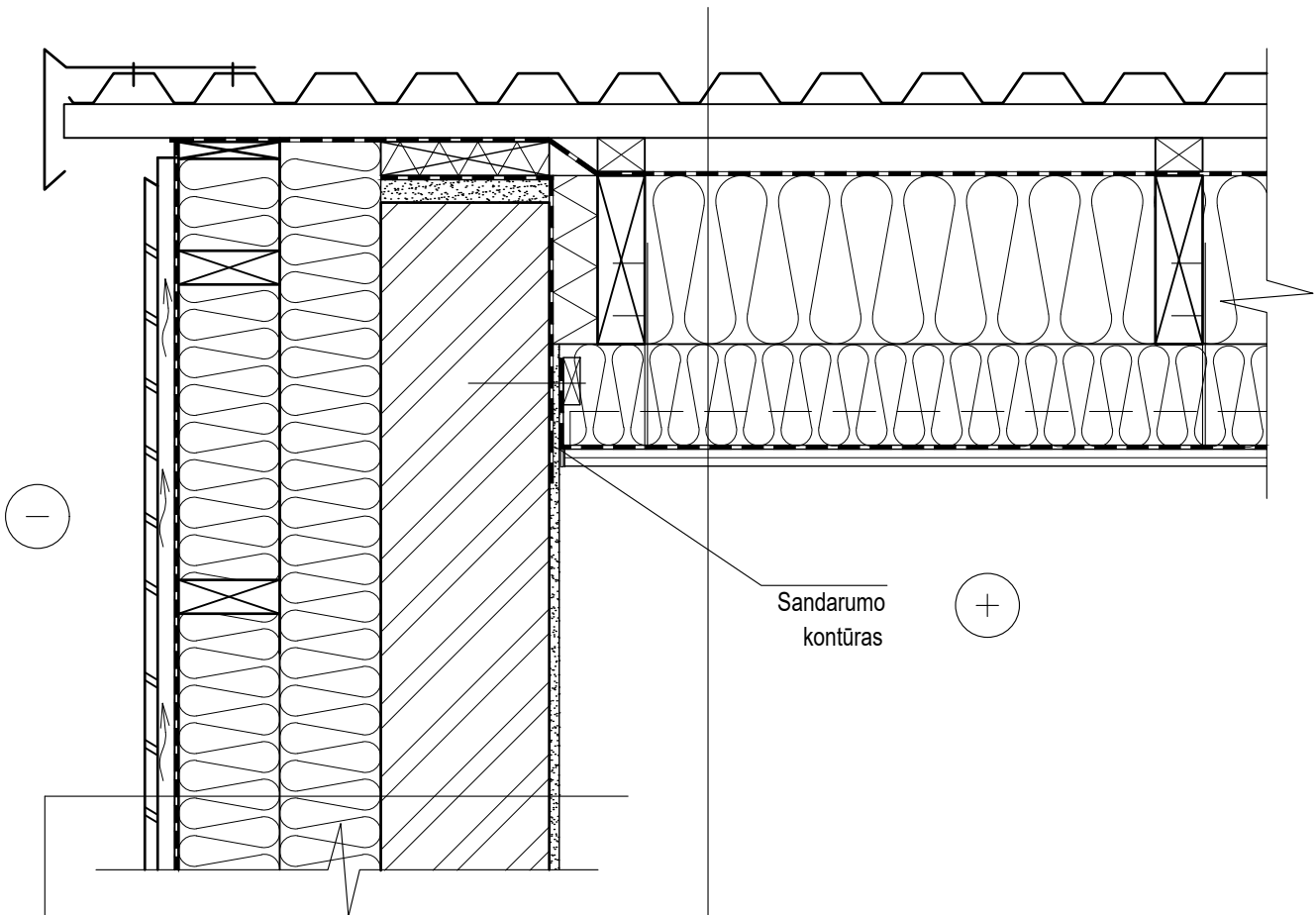
DET. "ST-1"
