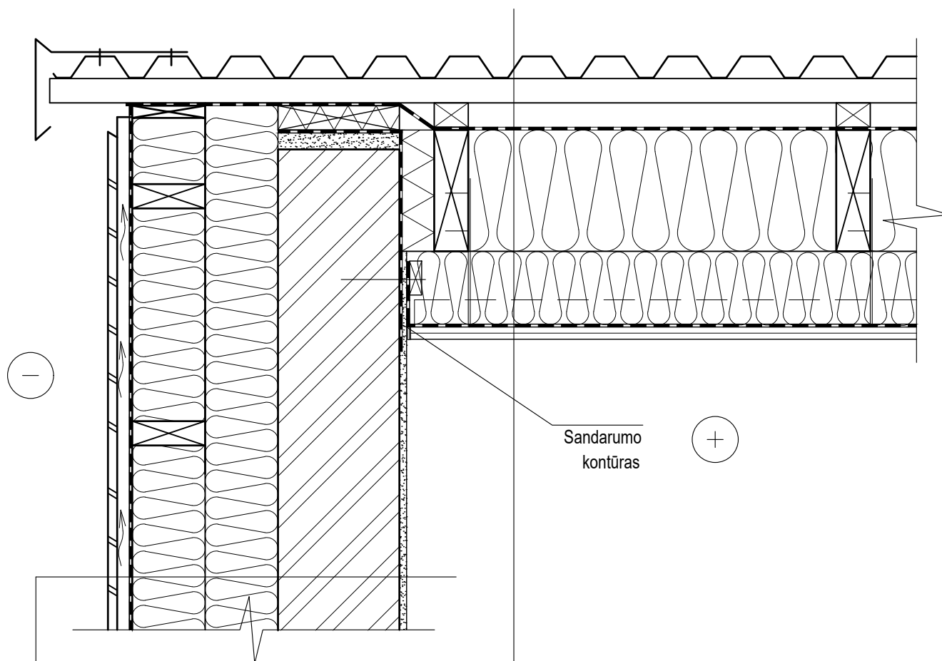
DET. "ST-1"
