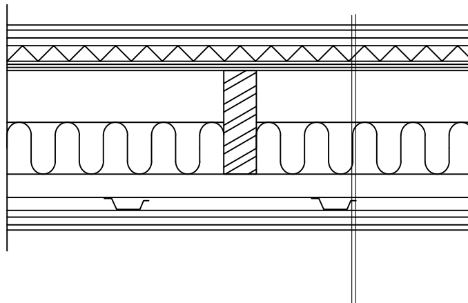
DET. "MP-5"
